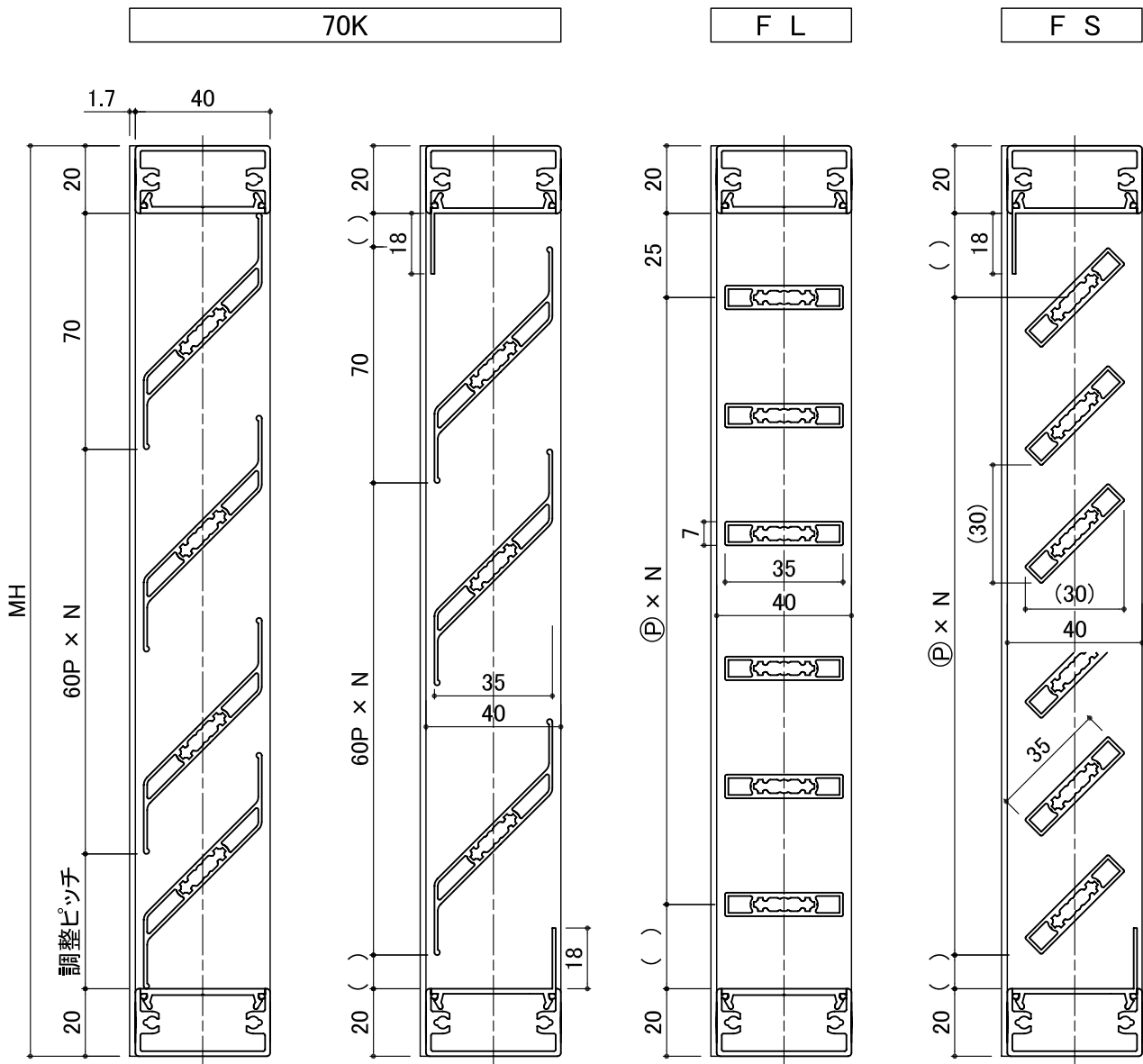
最下部羽根材による調整
