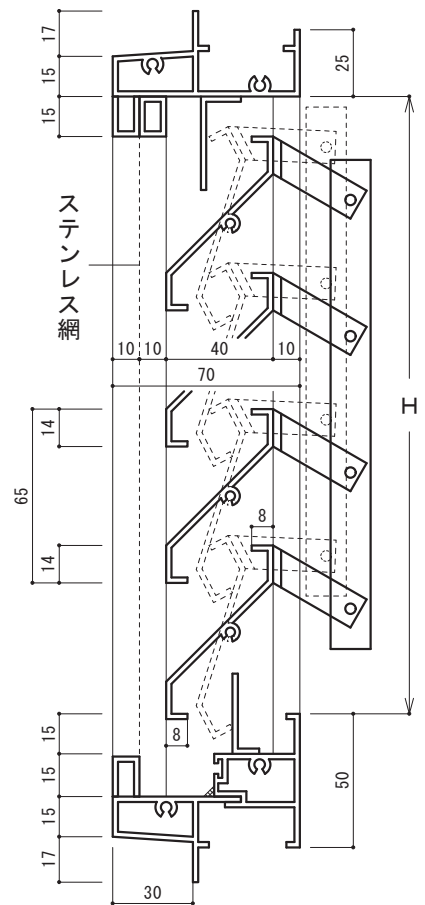
■半外付角可動ガラリ70枠網付 NO-9 1HKN
